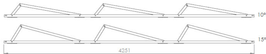
Variante 03: drei Dreiecksständer auf einer Grundschiene
